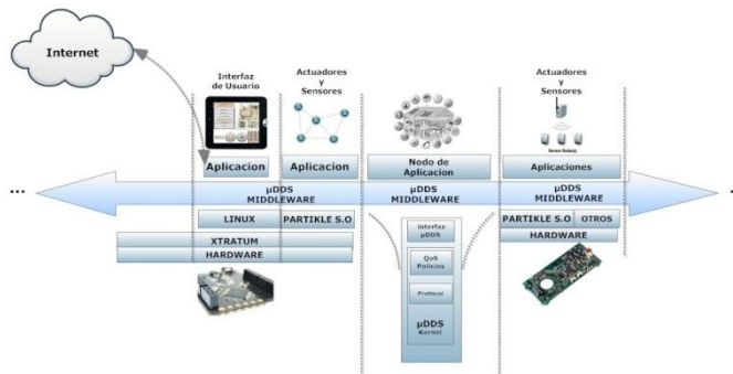
Fig. 5: Arquitectura de comunicaciones
