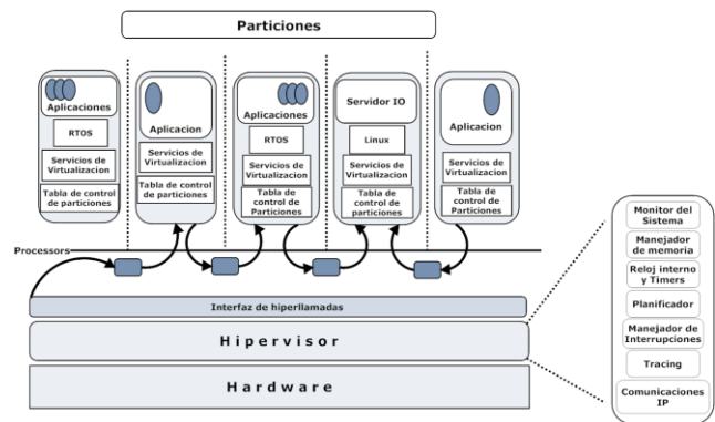
Fig. 4: Arquitectura interna de XtratuM
