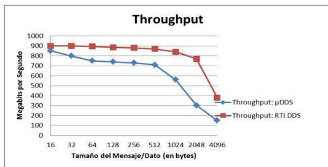
Fig. 7: Prueba de caudal Eficaz de la implementación \mu DDS.
